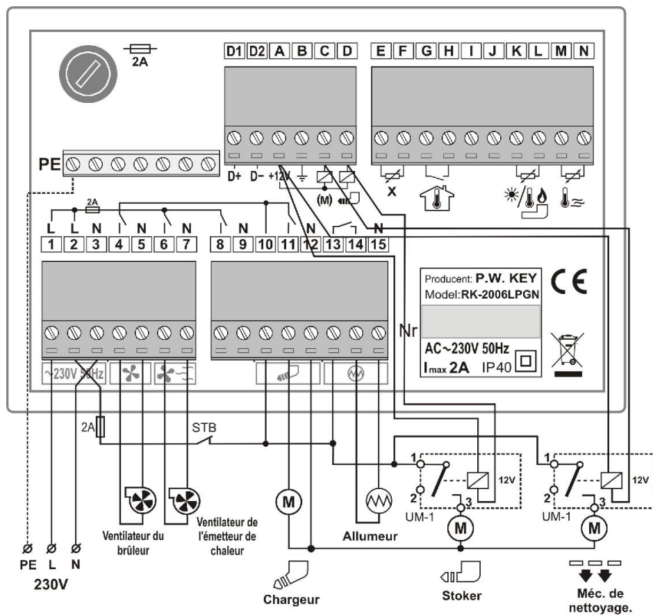
Figure 2. Schéma de câblage du régulateur RK-2006LPGN.
