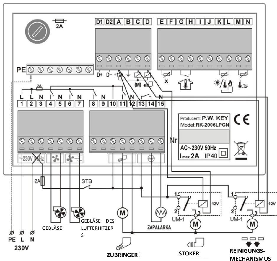
Abbildung 2. Anschlussschema des Reglers RK-2006LPGN.
