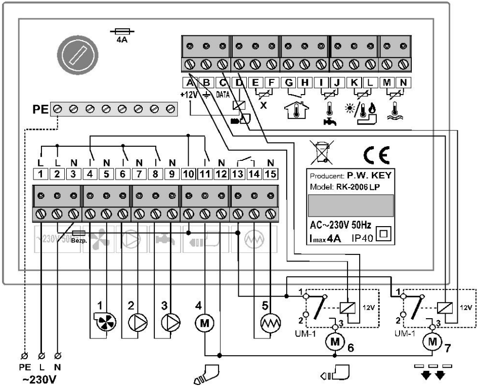
Abbildung 2. Schaltplan des Reglers RK-2006LP.
